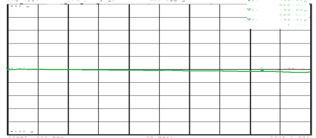
VSWR(input)
