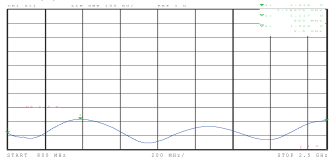
VSWR(in)
